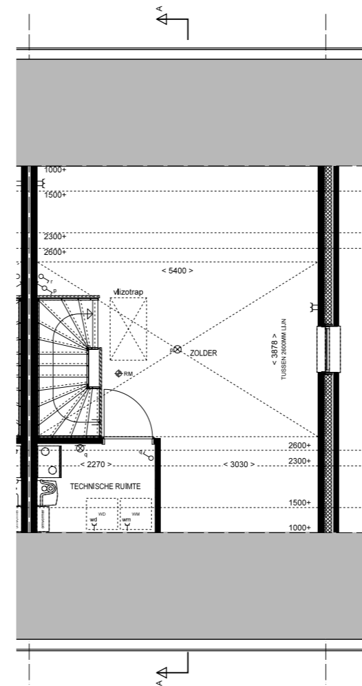
2e Verdieping 1:50 Bnr: 19 Type: A4
