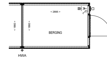
PLATTEGROND BERGING 1:50
