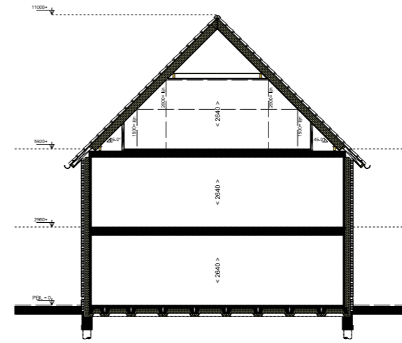
Doorsnede 1:100
