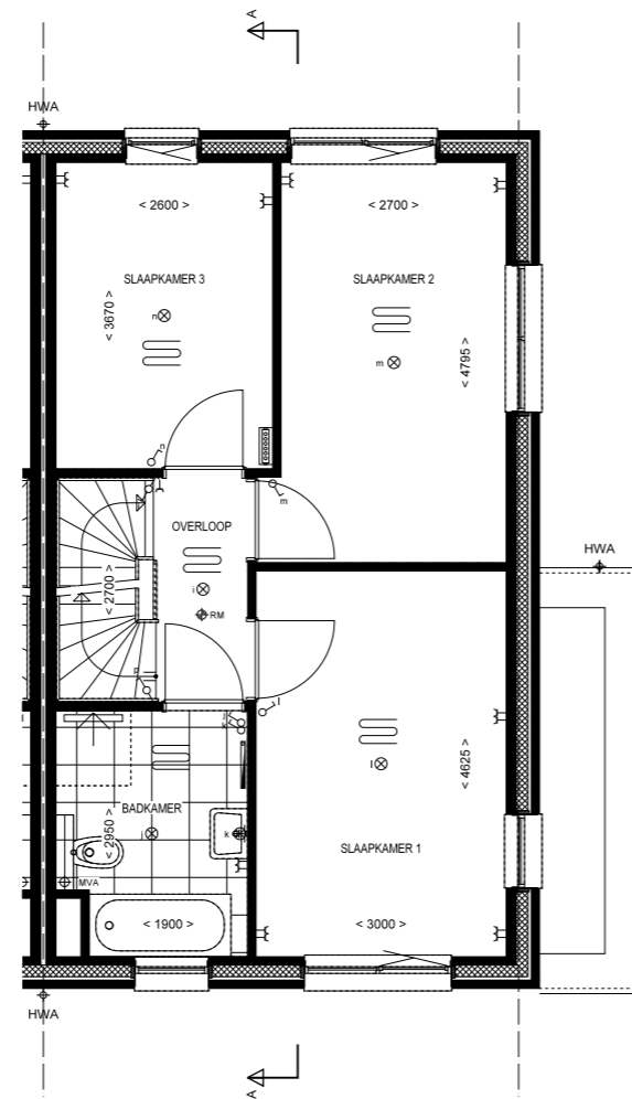
1e Verdieping 1:50 Bnr: 19 Type: A4
