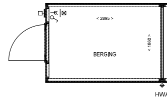
PLATTEGROND BERGING 1:50
