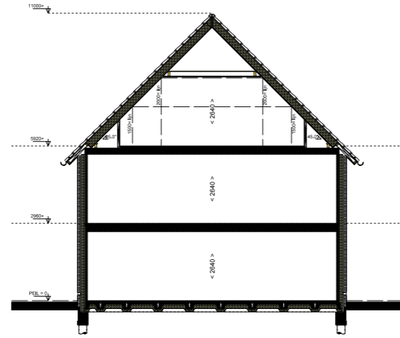
Doorsnede 1:100
