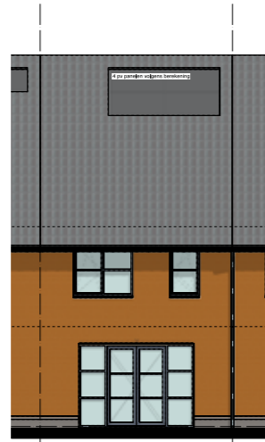
Achtergevel 1:100 Bnr: 21 Type: A2
