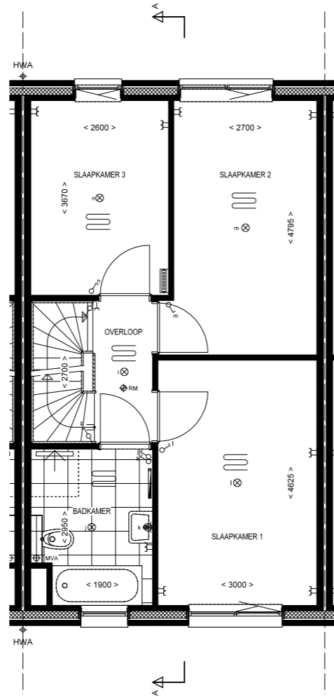
1e Verdieping 1:50 Bnr: 21 Type: A2
