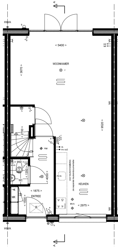
Begane grond 1:50 Bnr: 21 Type: A2
