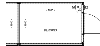
PLATTEGROND BERGING 1:50
