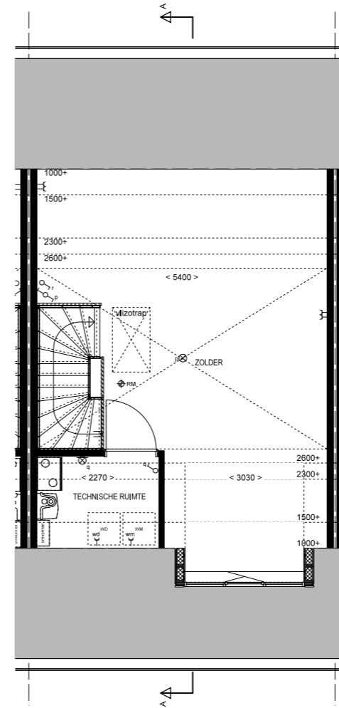
2e Verdieping 1:50 Bnr: 21 Type: A2
