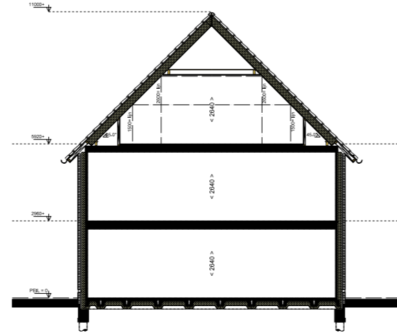
Doorsnede 1:100
