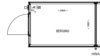
PLATTEGROND BERGING 1:50
