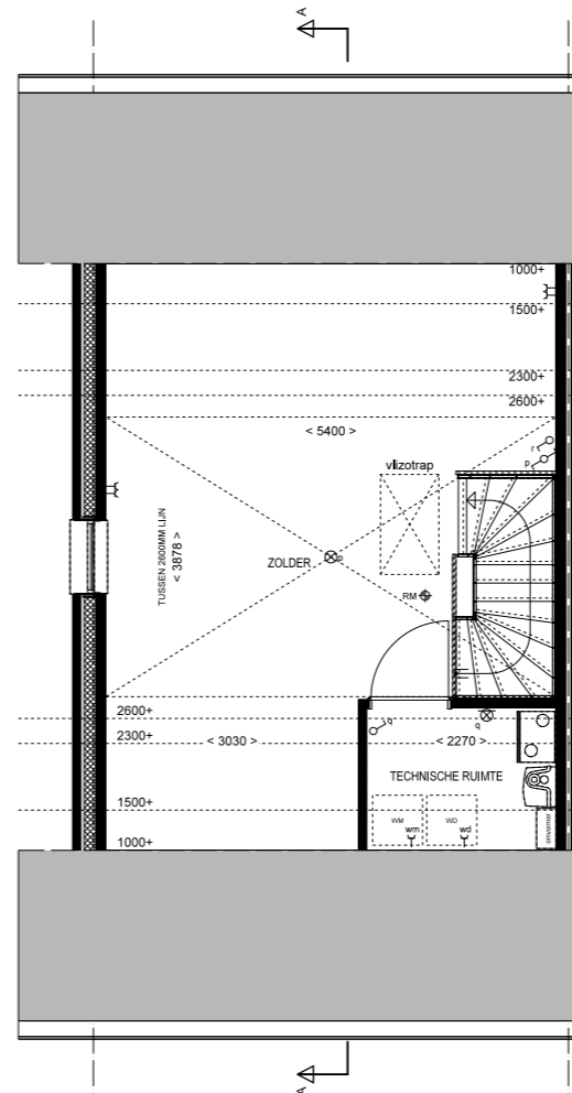
2e Verdieping 1:50 Bnr: 22 Type: A3sp
