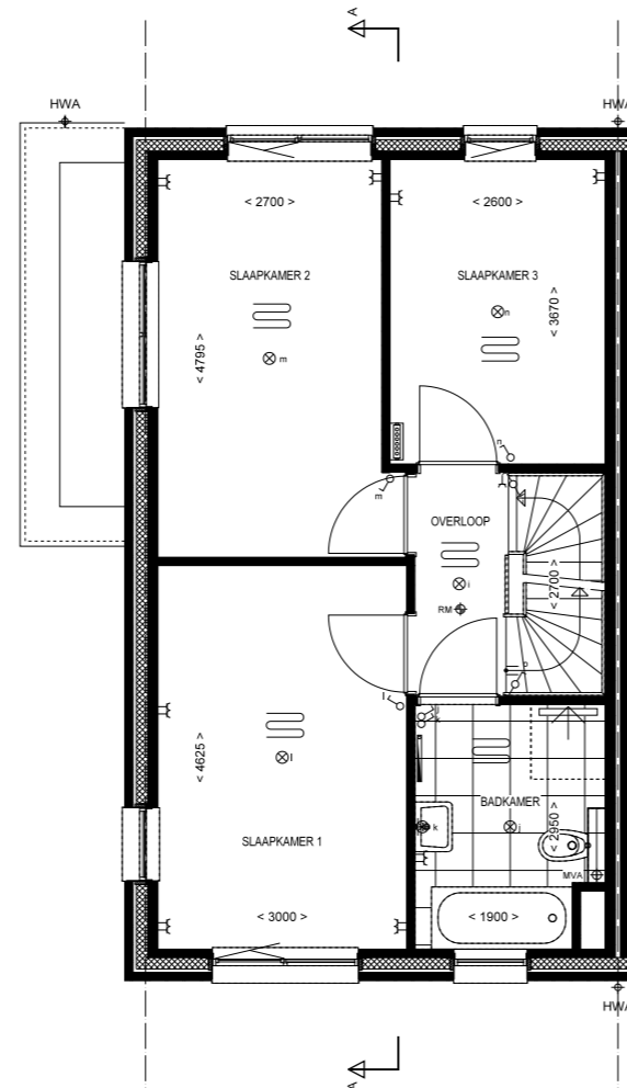
1e Verdieping 1:50 Bnr: 22 Type: A3sp
