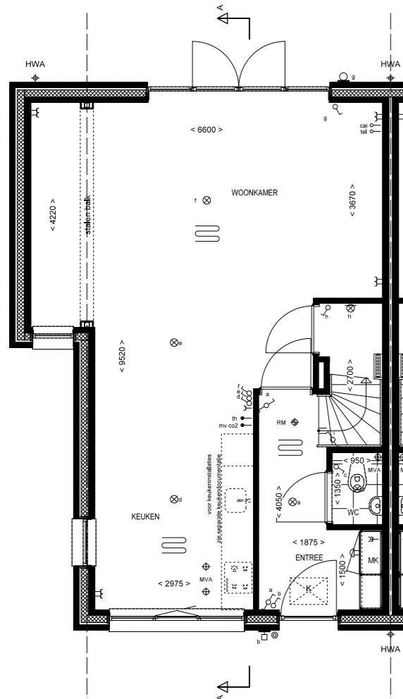
Begane grond 1:50 Bnr: 22 Type: A3sp
