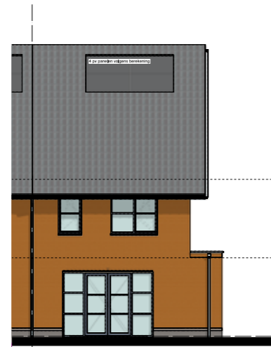
Achtergevel 1:100 Bnr: 22 Type: A3sp
