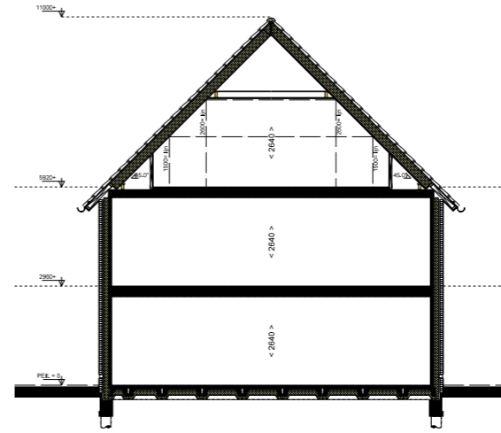
Doorsnede 1:100
