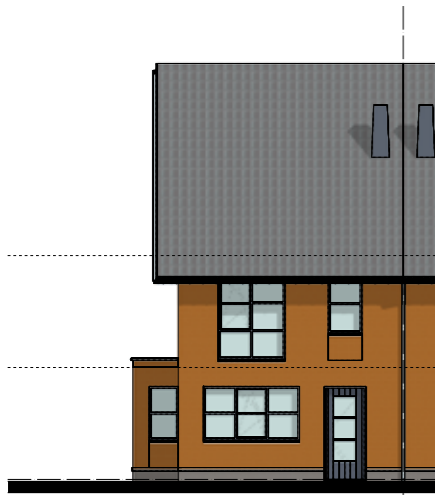
Voorgevel 1:100 Bnr: 22 Type: A3sp
