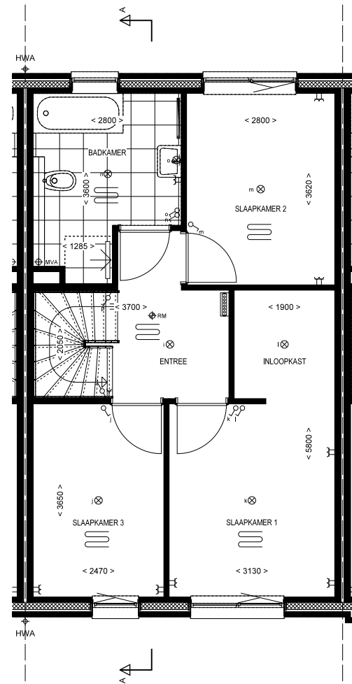
1e Verdieping 1:50 Bnr: 24 Type: B2
