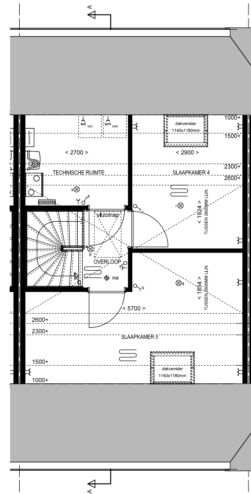
2e Verdieping 1:50 Bnr: 24 Type: B2
