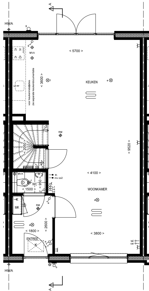
Begane grond 1:50 Bnr: 24 Type: B2
