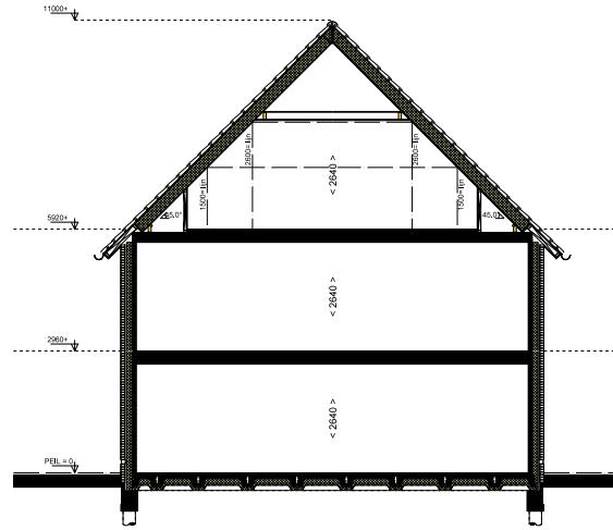
Doorsnede 1:100
