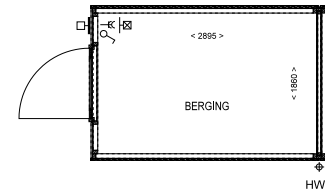
PLATTEGROND BERGING 1:50
