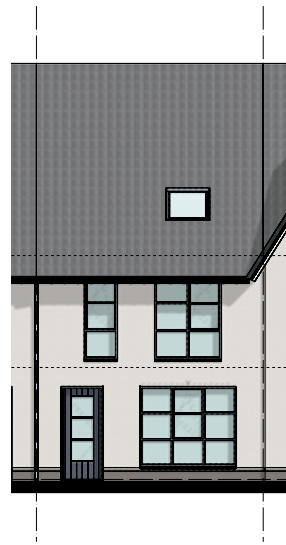
Voorgevel 1:100 Bnr: 24 Type: B2
