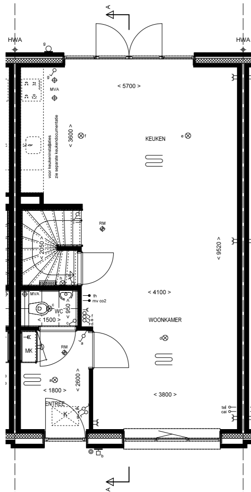
Begane grond 1:50 Bnr. 26 Type: B3
