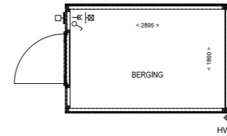
PLATTEGROND BERGING 1:50
