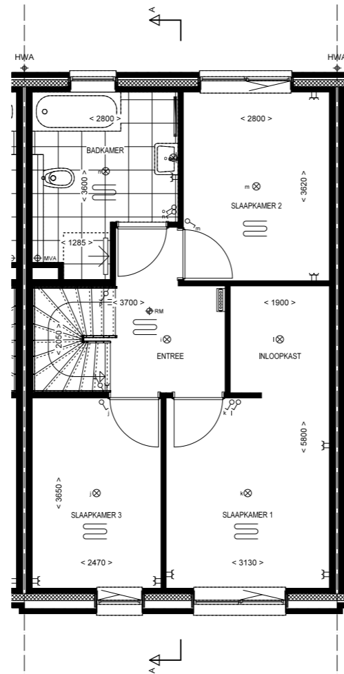
1e Verdieping 1:50 Bnr. 26 Type: B3
