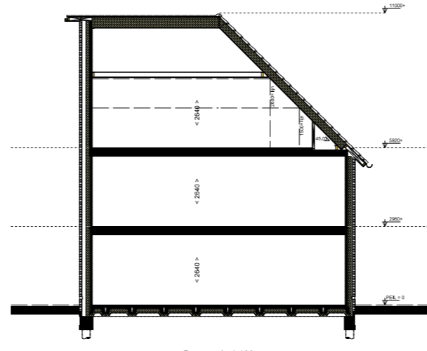
Doorsnede 1:100
