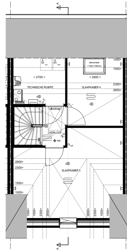
2e Verdieping 1:50 Bnr. 26 Type: B3
