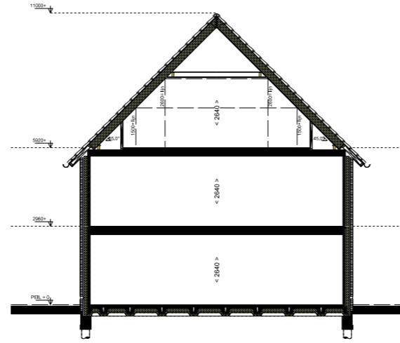
Doorsnede 1:100
