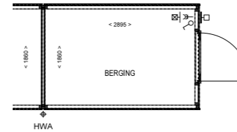
PLATTEGROND BERGING 1:50
