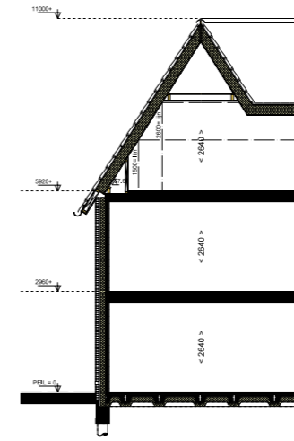
Doorsnede 1:100
