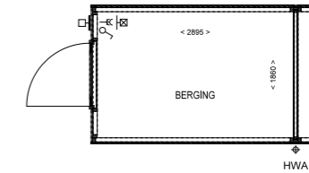
PLATTEGROND BERGING 1:50
