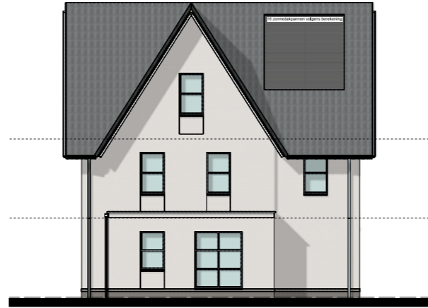
Linker zijgevel 1:100 Bnr: 28 Type: B6sp
