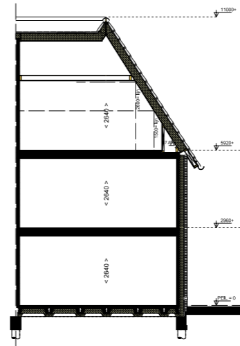
Doorsnede 1:100
