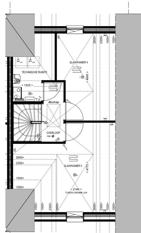
2e Verdieping 1:50
