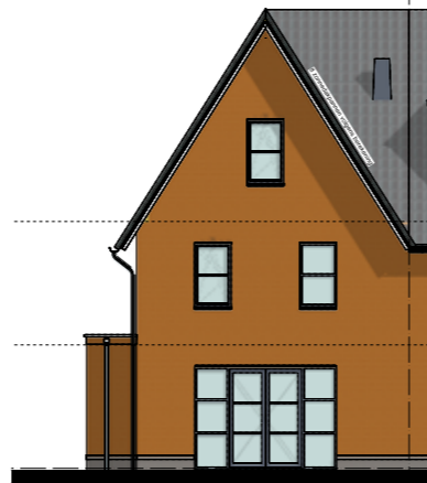
Achtergevel 1:100 Bnr: 29 Type: C9
