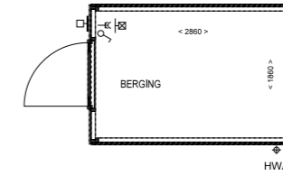
PLATTEGROND BERGING
