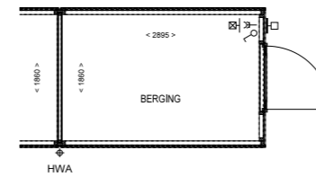
PLATTEGROND BERGING 1:50
