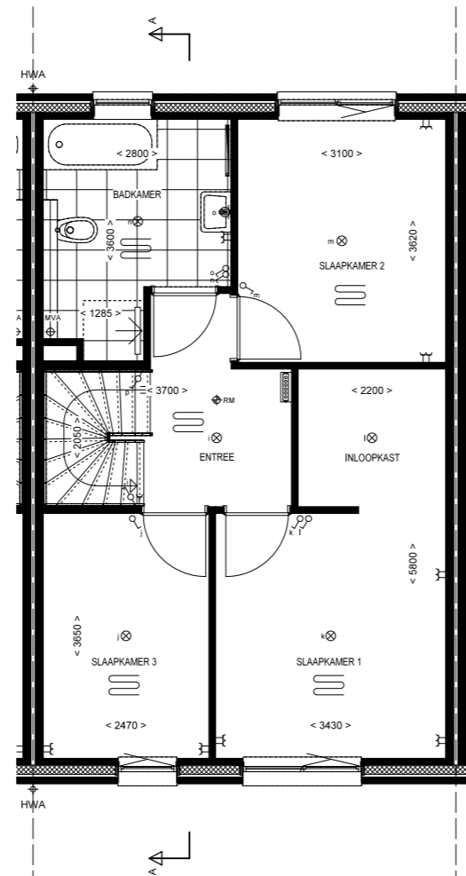
1e Verdieping 1:50 Bnr: 30 Type: C7
