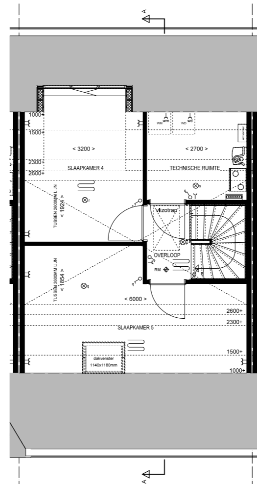
2e verdieping 1:50 Bnr: 31 Type: C7sp
