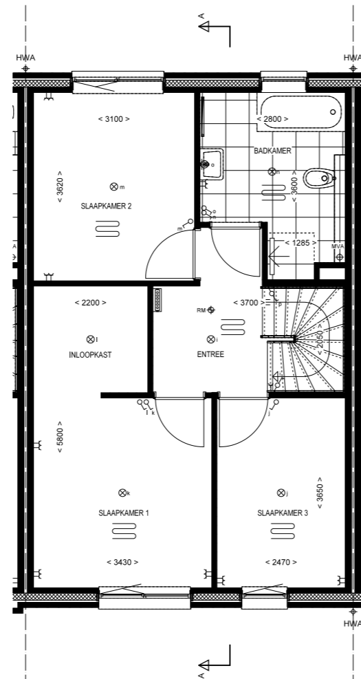
1e verdieping 1:50 Bnr: 31 Type: C7sp
