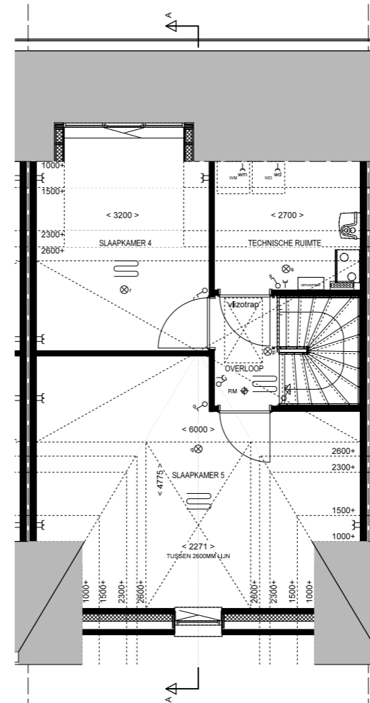
2e Verdieping 1:50 Bnr: 32 Type: C8sp
