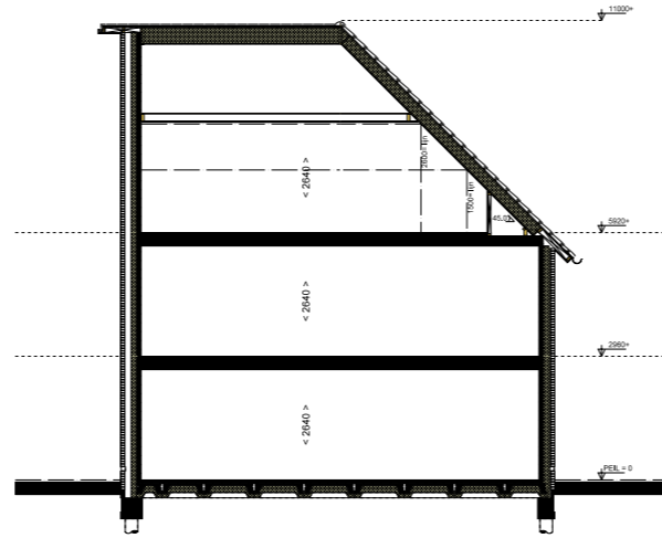
Doorsnede 1:100
