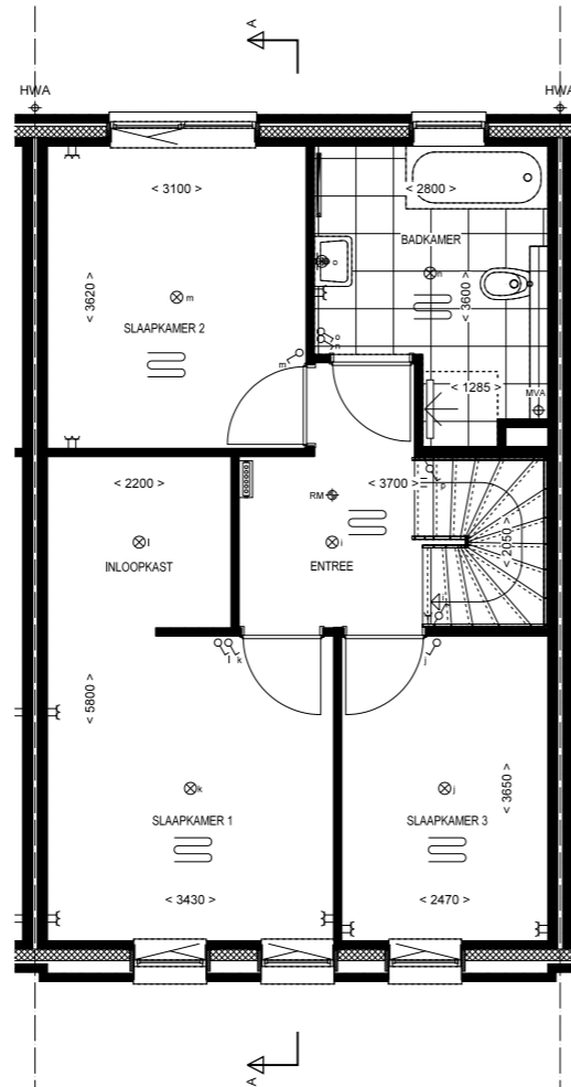
1e Verdieping 1:50 Bnr: 32 Type: C8sp
