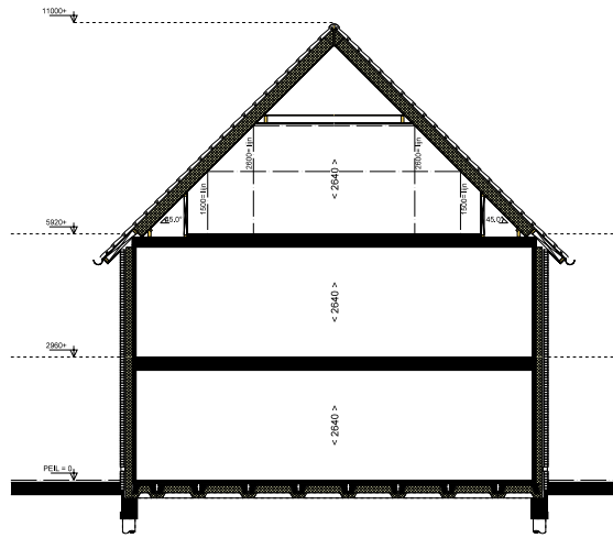
Doorsnede 1:100
