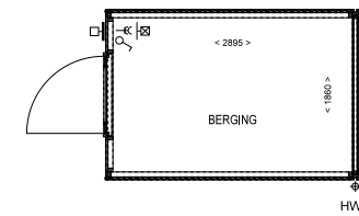
PLATTEGROND BERGING 1:50
