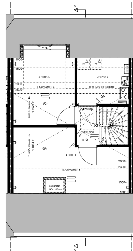
2e Verdieping 1:50 Bnr: 34 Type: C7sp
