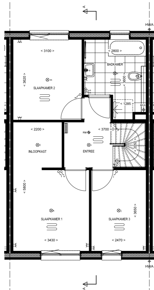
1e Verdieping 1:50 Bnr: 34 Type: C7sp
