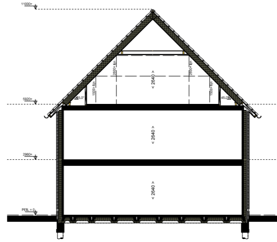
Doorsnede 1:100
