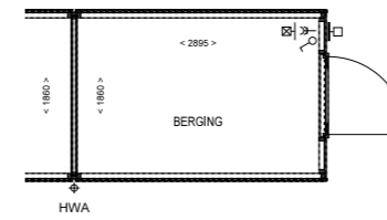
PLATTEGROND BERGING 1:50
