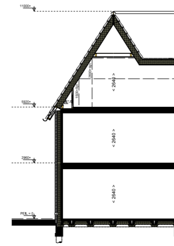
Doorsnede 1:100
