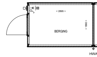
PLATTEGROND BERGING 1:50
