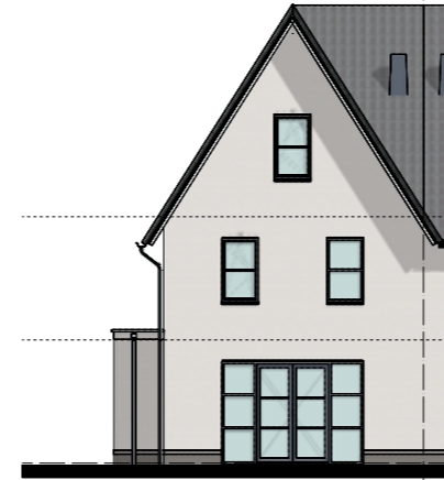
Voorgevel 1:100 Bnr. 36 Type: B8
