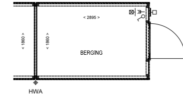
PLATTEGROND BERGING 1:50
