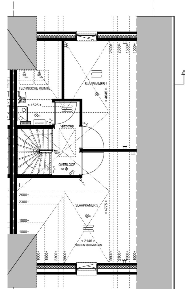
2e Verdieping 1:50 Bnr. 36 Type: B8
