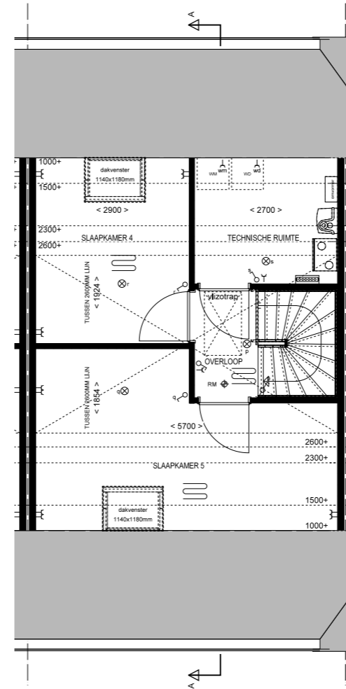
2e Verdieping 1:50 Bnr: 37 Type: B7sp
