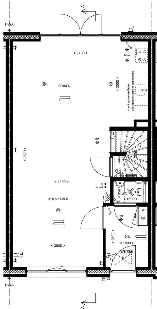
Begane grond 1:50 Bnr: 37 Type: B7sp
