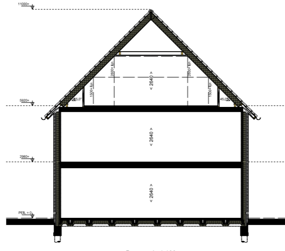
Doorsnede 1:100
